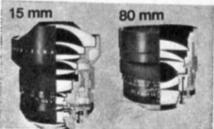
ФОТО 7. НОВЫЕ ОБЪЕКТИВЫ «ЛЕЙКИ R4»
