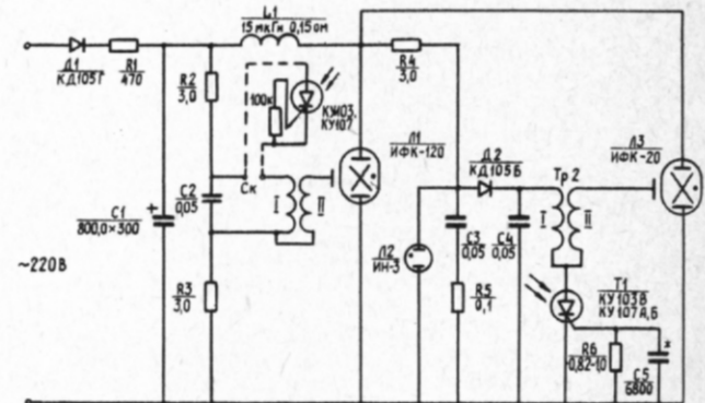
РИС. 1. ПРИНЦИПИАЛЬНАЯ СХЕМА АВТОМАТИЧЕСКОЙ ШУНТОВОЙ ФОТОВСПЫШКИ
